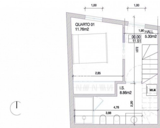
PLANTA PISO 0
